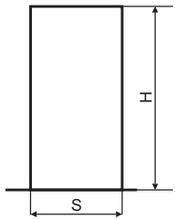
Dimensions of holes in the wall for Arcus door frame assembly Размеры дверного проема для установки коробки Arcus Dimensions [mm] / Размеры [mm]
