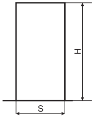
Door-way dimensions for adjustable door frame assembly Размеры дверного проема в стене для установки регулируемой коробки Dimensions [mm] / Размеры [мм]
