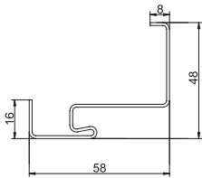
BORD corner steel door-frame Коробка BORD СТАЛЬНАЯ угловая
