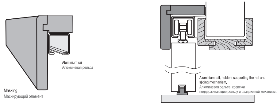
Vertical cross-section of sliding system Вертикальный разрез раздвижной системы
