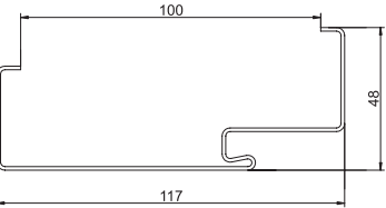
BORD fixed door-frame Коробка BORD СТАЛЬНАЯ
